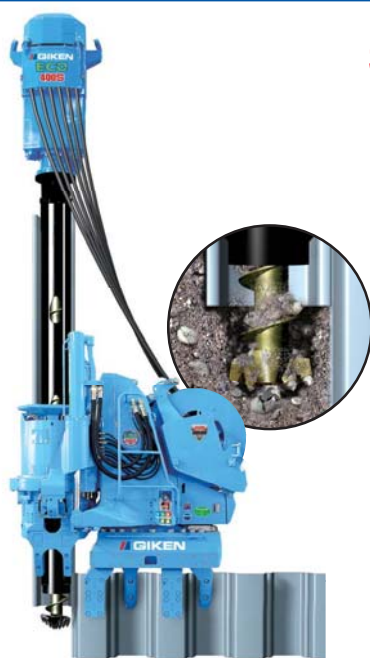
硬質地盤圧入時
